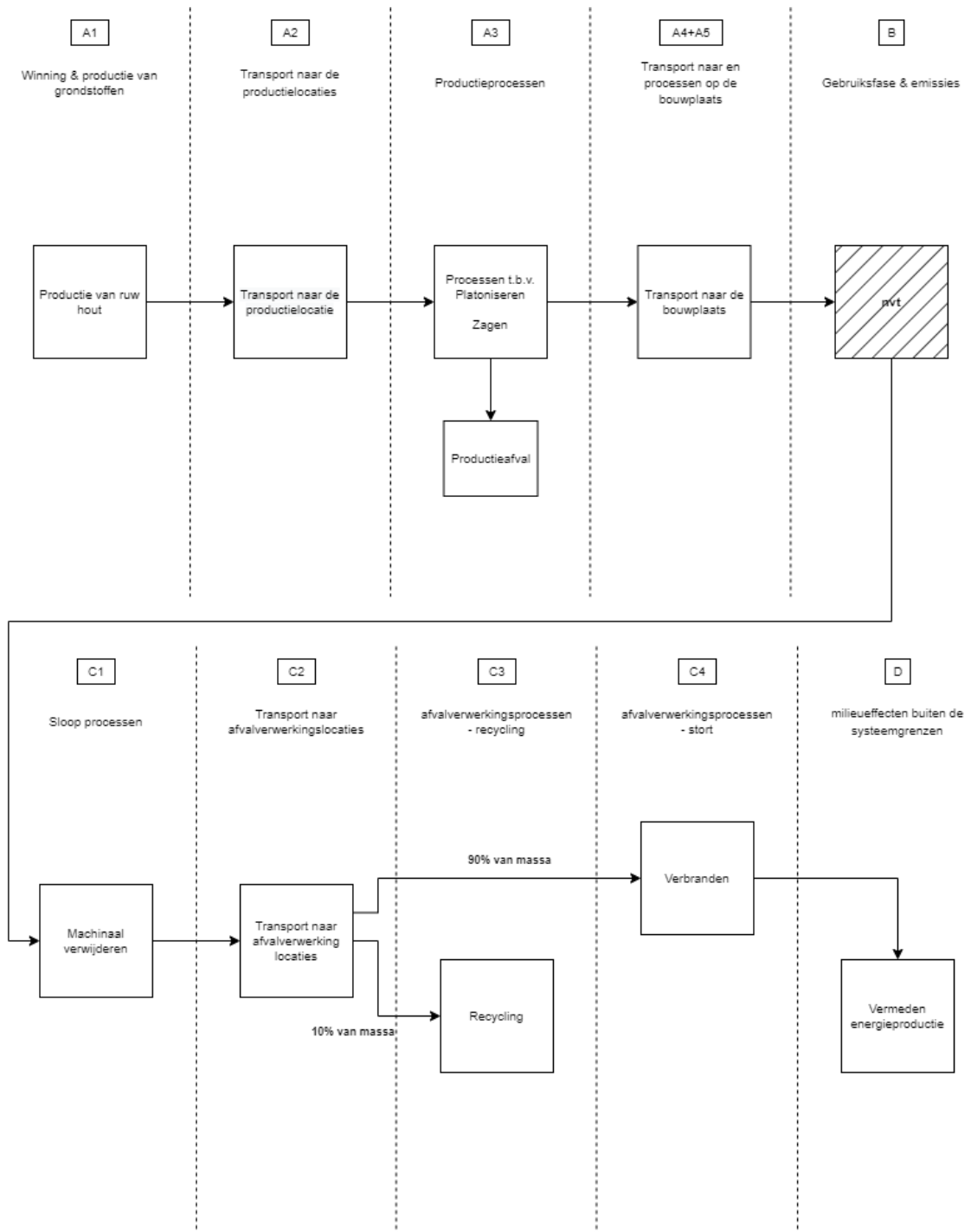
LCA proces diagram volgens EN 15804 (7.2.1)
